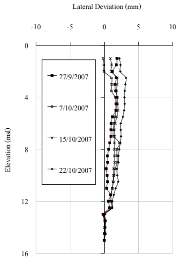
ภาพที่ 10 การเคลื่อนตัวด้านข้างในแนวความลาดเอียง ตำแหน่งที่ 2
