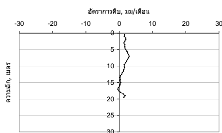
ภาพที่ 9 อัตราการเคลื่อนตัวตามความลึก ตำแหน่งที่ 1
