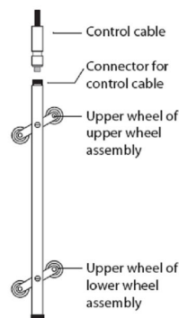
Digitilt Inclinometer
