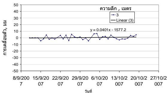
ภาพที่ 6 ตัวอย่างการคำนวณอัตราการคืบของลาดดินด้านข้างในแนวความลาดเอียง โดยวิธี Regression analysis
