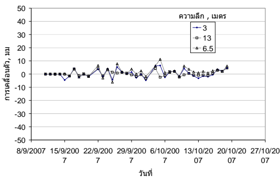
ภาพที่ 5 การเคลื่อนตัวด้านข้างในแนวความลาดเอียง ตามระยะเวลา ตำแหน่งที่ 1
