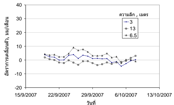
ภาพที่ 7 อัตราการเคลื่อนตัวตามระยะเวลา ตำแหน่งที่ 1
