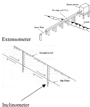
ภาพที่ 1 เครื่องมือวัดการเคลื่อนตัวรูปแบบต่างๆ
