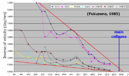
ภาพที่ 15 ตัวอย่างการเตือนภัยโดยใช้การเคลื่อนตัวในประเทศอิตาลี [5]
