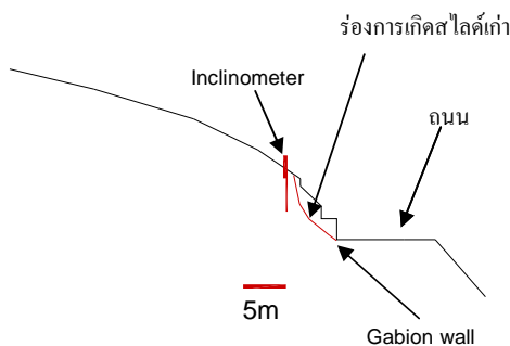
ภาพที่ 13 การติดตั้ง In Place Inclinerometer ตำแหน่งที่ 3
