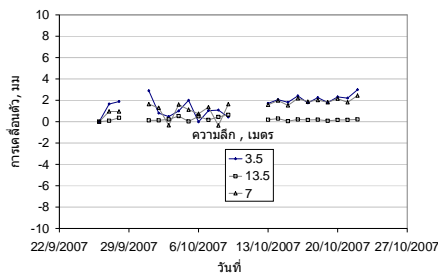
ภาพที่ 11 การเคลื่อนตัวด้านข้างในแนวความลาดเอียง ที่ความลึกต่างกัน ตำแหน่งที่ 2
