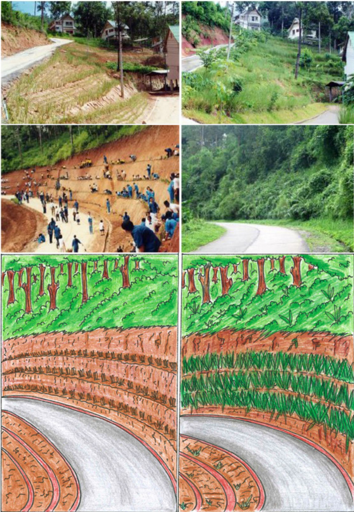
รูปที่ 10 การประยุกต์ใช้หญ้าแฝกเพื่อแก้ไขดินถล่มในพื้นที่ต่าง ๆ ในประเทศไทย ภาพระหว่างปลูก และหลังปลูก เมื่อหญ้าแฝกโต (ดร.วีระชัย ณ นคร เอื้อเฟื้อรูปประกอบ)
