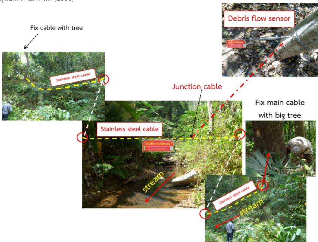
รูปที่ 28 ตัวอย่างขั้นตอนการติดตั้งเครื่องมือตรวจวัดการไหล (debris flow sensor) ในพื้นที่เสี่ยงภัยดินถล่มและน้ำป่าไหลหลาก
