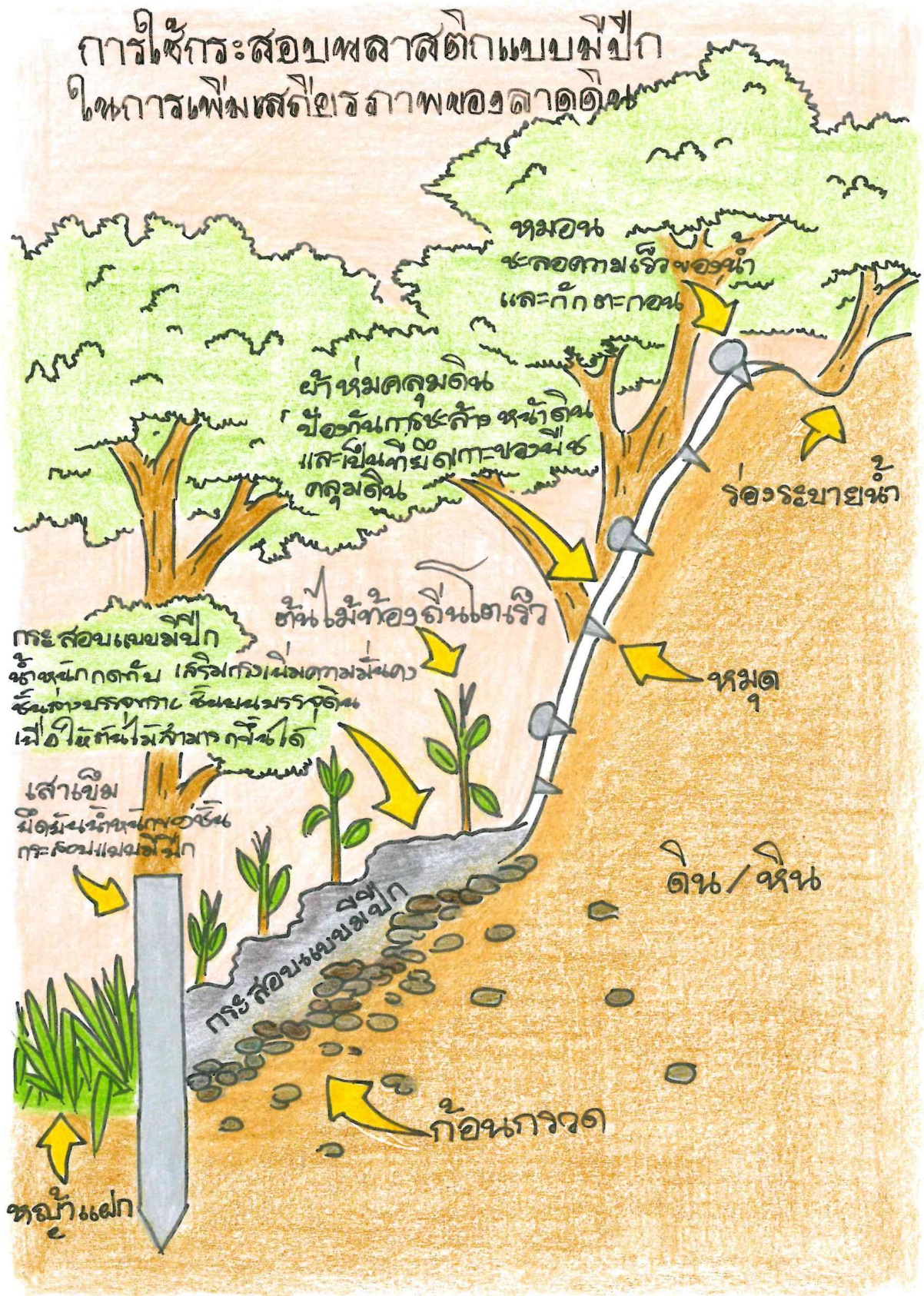
รูปที่ 11 รูปแบบการเรียงกระสอบมีปีกผสมผสานกับวิธีทางวิศวกรรมและการใช้พืชต่างๆเพื่อเสริมเสถียรภาพของลาด ที่มา : ดัดแปลงรูปจาก บริษัท พีทีที โกลบอลเคมิคอล จำกัด (มหาชน)
