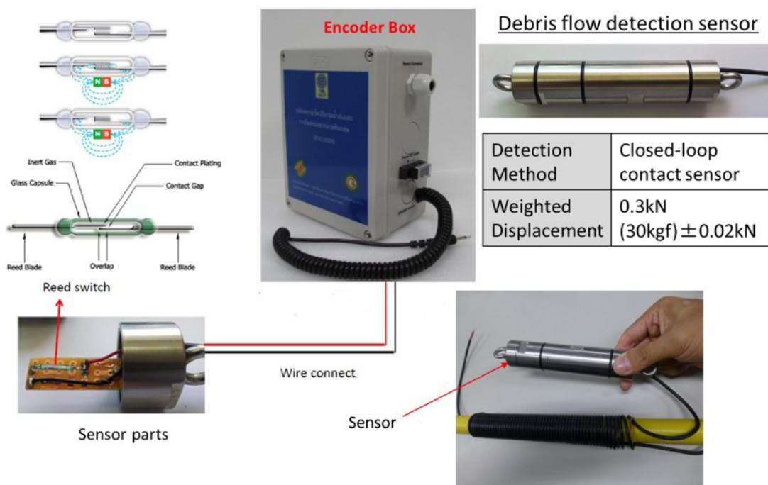
รูปที่ 24 อุปกรณ์ตรวจวัดการไหลดินถล่ม debris flow detector sensor
