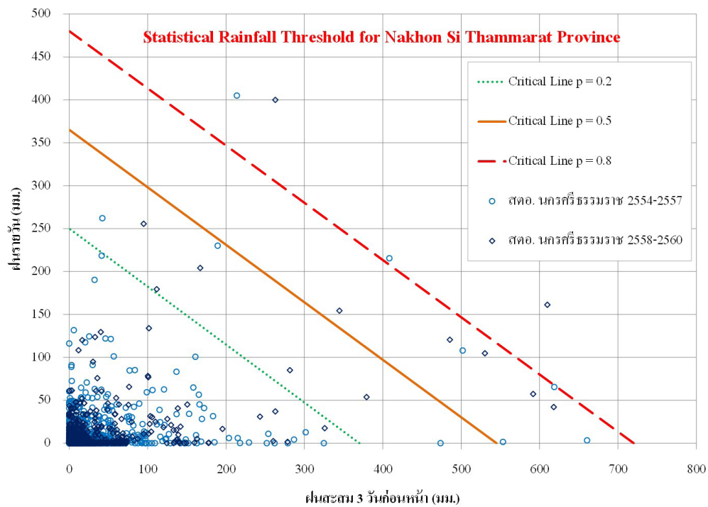
รูปที่ 33 ตัวอย่างการสร้างเกณฑ์ปริมาณน้ำฝนวิกฤติเชิงสถิติของพื้นที่ภาคใต้ฝั่งตะวันออก (ข้อมูลน้ำฝนจากสถานีอุตุนิยมวิทยาจังหวัดนครศรีธรรมราช (พ.ศ. 2554-2560))
