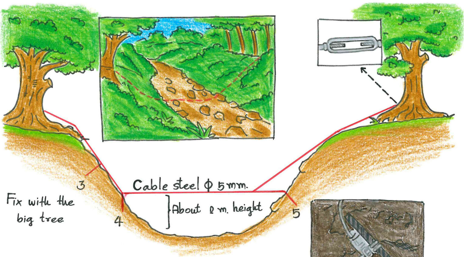
รูปที่ 27 ตัวอย่างการติดตั้งเครื่องมือตรวจวัดการไหล (debris flow sensor)
